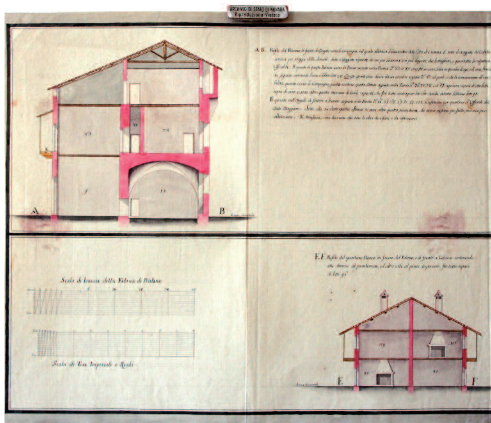
Tav. X - Sezioni AB ed EF del castello di Cremona, XVIII sec. Archivio di Stato di Novara (Scheda 40)
