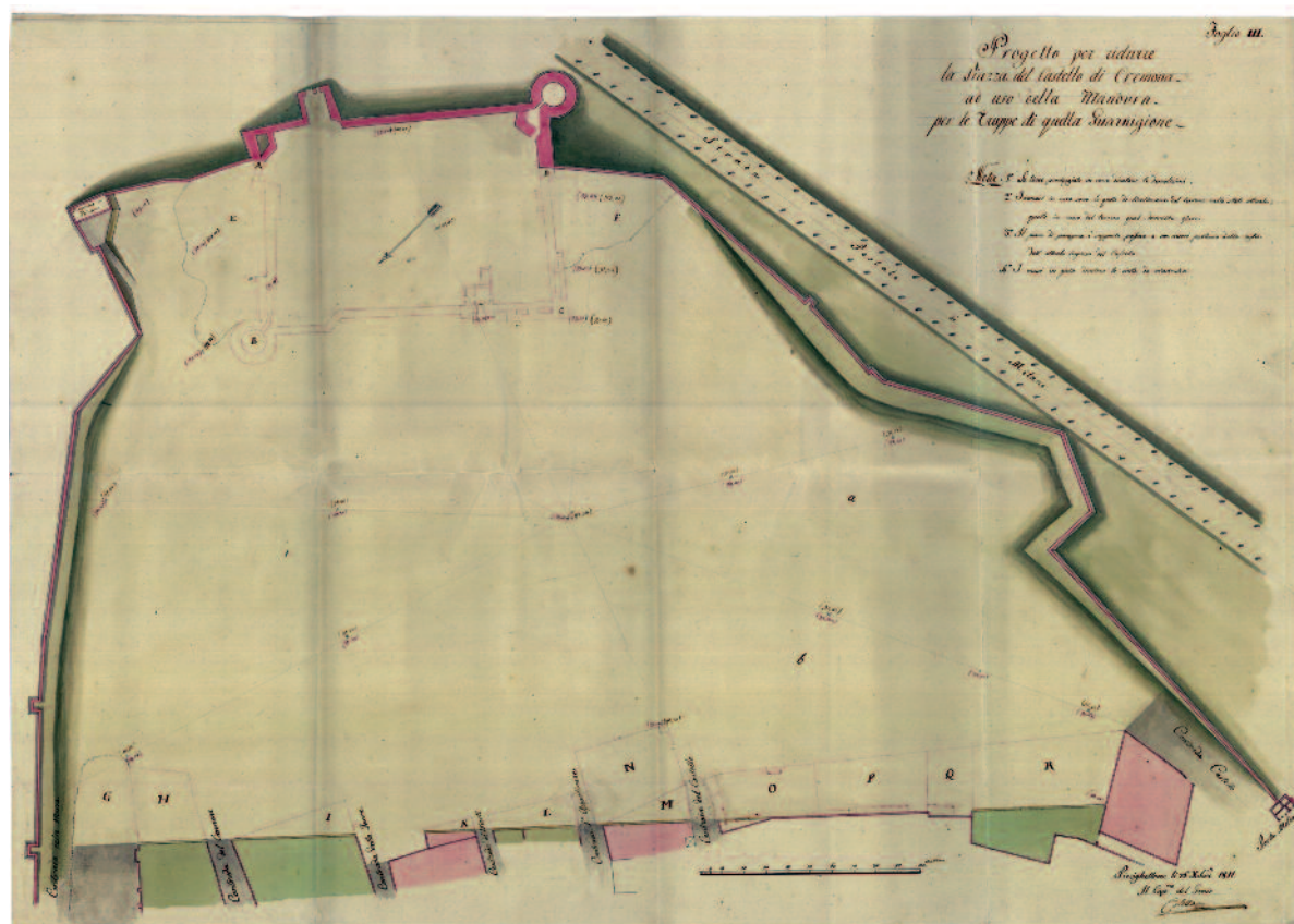
Tav. XV - Colella, Progetto per ridurre la Piazza del Castello di Cremona ad uso della Manovra per le Truppe di quella Guarnigione , 1811. Archivio di Stato di Milano (Scheda 49)
