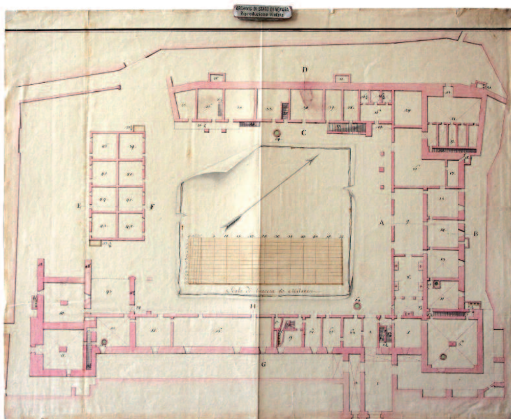
Tav. VIII - Pianta del piano terreno del castello di Cremona, XVIII sec. Archivio di Stato di Novara (Scheda 38)
